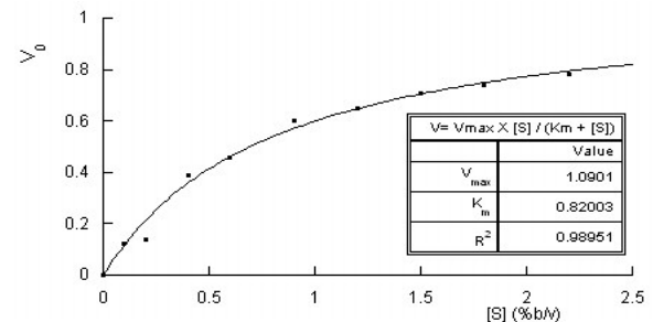
Gambar 4. Kurva V 0 vs [S] berdasarkan persamaan Michaelis-Menten
