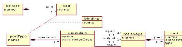
Struktur definisi WSDL dalam model UML
