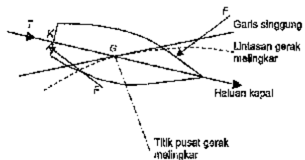
Gambar 3. Gaya-gaya yang bekerja dalam proses setting pada saat manover
