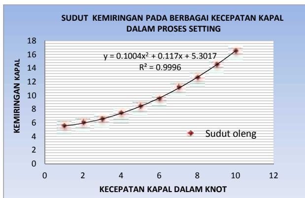
Gambar 9 Grafik hubungan kecepatan dengan kemiringan kapal dalam proses setting
