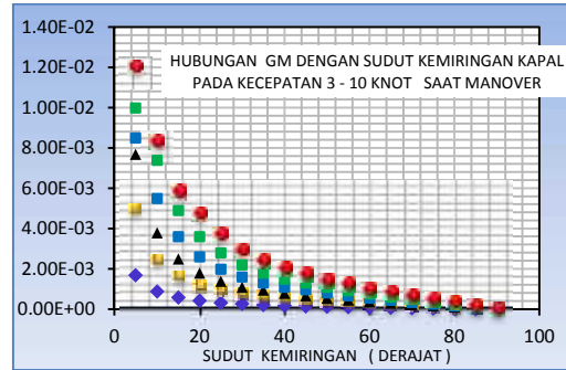
Gambar 7. Kurva GM pada saat Manover
