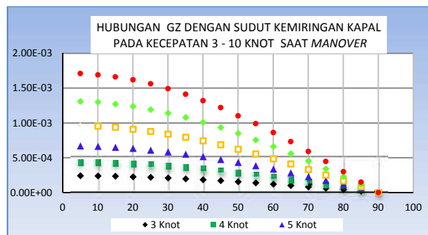
Gambar 8. Kurva GZ pada saat Manover
