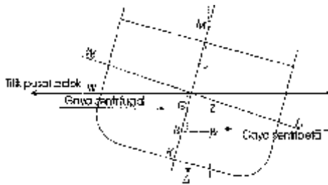
Gambar 4. Gaya-gaya yang bekerja pada saat manover dalam proses setting
