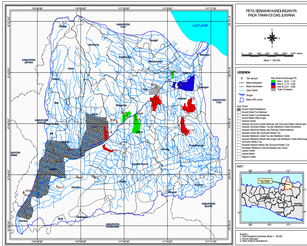
Gambar 1. Sebaran logam Pb pada tanah sawah Sub-DAS Juwana
